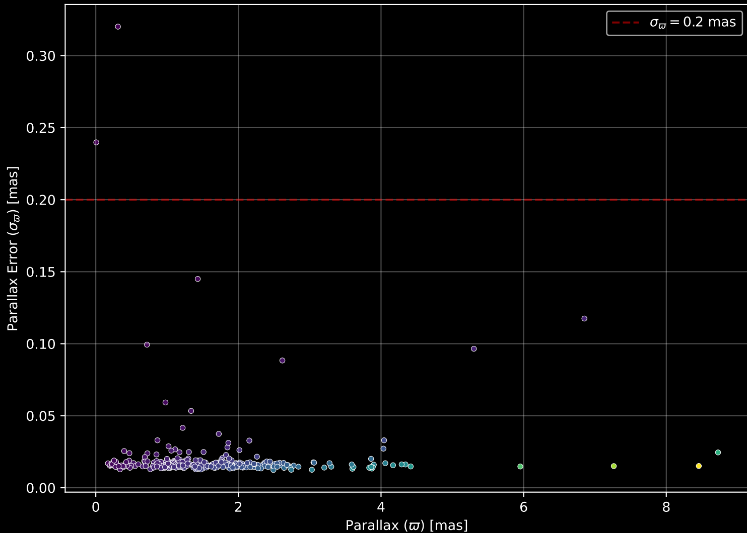
GALAH DR4 Field: [1467] Parallax Quality (n= 273)
