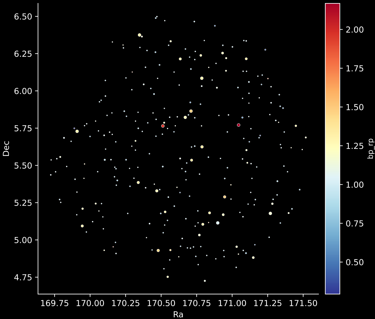
GALAH DR4 Field: [1467] Stars: 273
