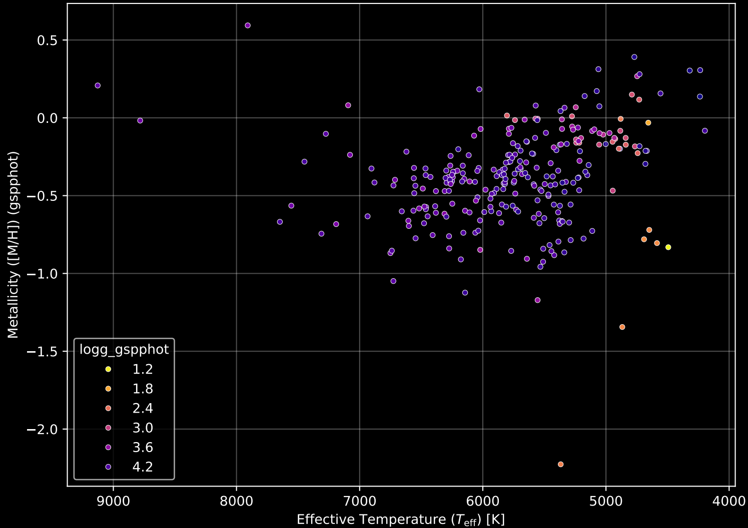
GALAH DR4 Field: [1467] Stellar Population Parameters (n= 273)
