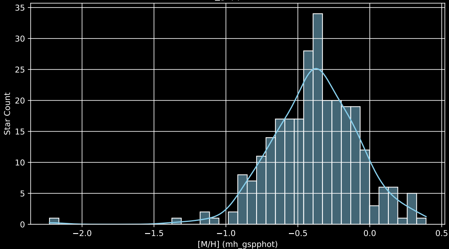
GALAH DR4 Field: [1467] [M/H] (mh_gspphot) (n= 272)
